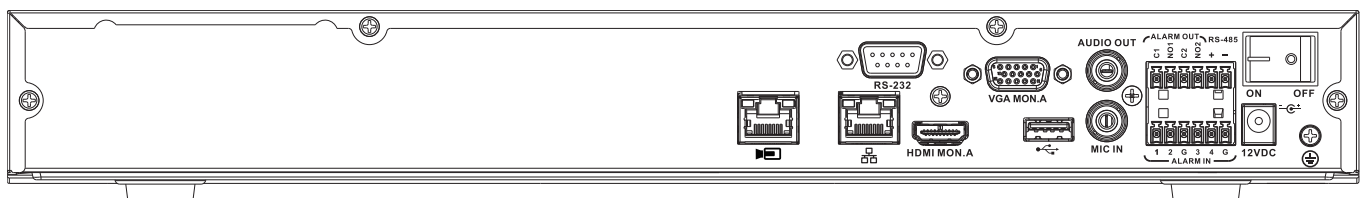
图片 1: DIVAR 3000网络后面板 (无PoE)
