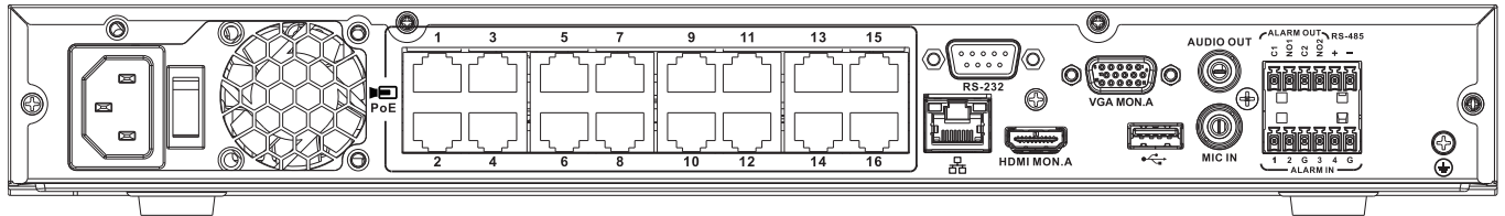
图片 2: DIVAR 3000网络后面板(16 PoE)
