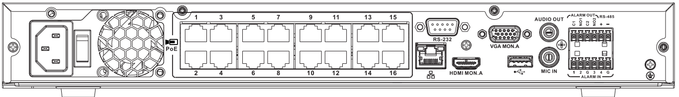
Şek. 2: DIVAR 3000 network arka panel (16 PoE)
