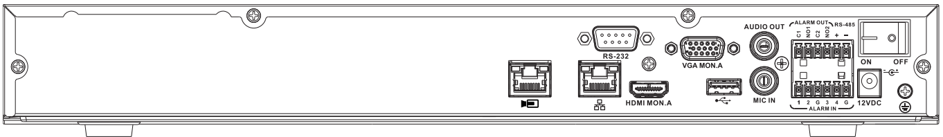
Fig. 1: Painel traseiro do DIVAR 3000 network (sem PoE)
