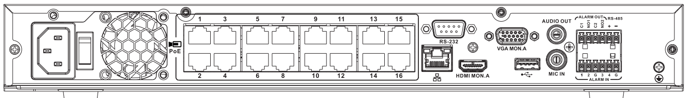
圖 3: DIVAR network 2000 (16 PoE) 後方面板
