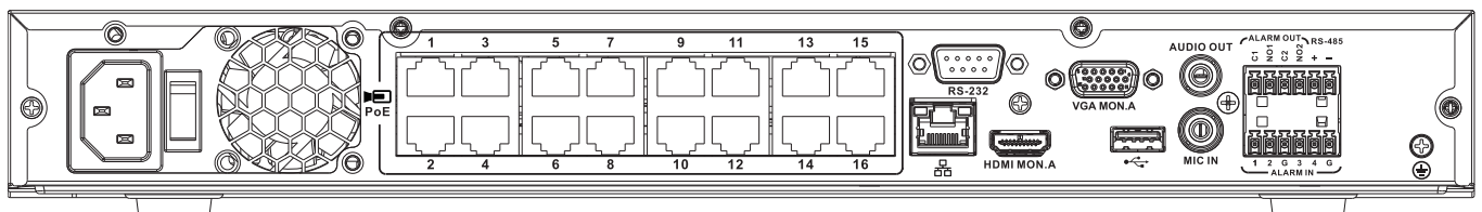
图片 3: DIVAR2000网络(16 PoE)后面板
