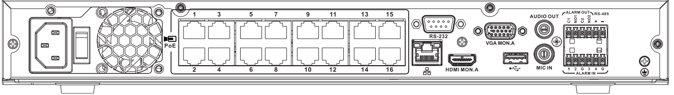
Şek. 3: DIVAR network 2000 (16 PoE) arka panel
