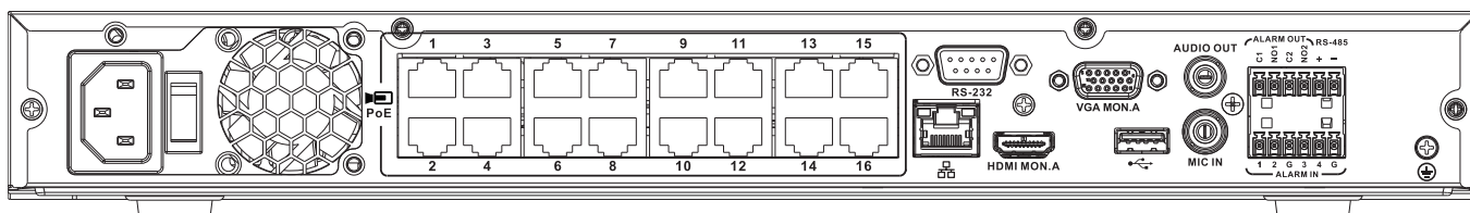
Рис. 3: Задняя панель DIVAR network 2000 (16 PoE)
