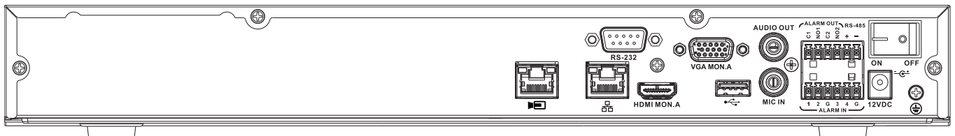
Рис. 1: Задняя панель DIVAR network 2000 (без PoE)
