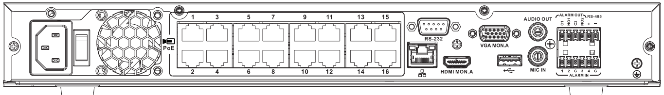
Fig. 3: DIVAR network 2000 (16 PoE), pannello posteriore
