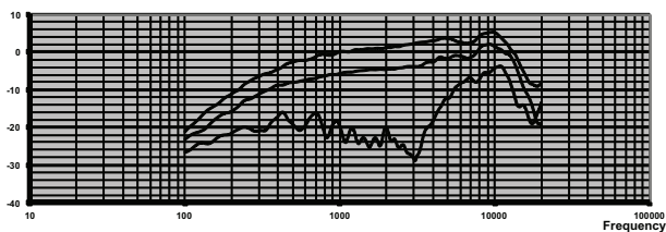
圖 1: 頻率響應 (開啟角度: 0、90 和 180 度)
