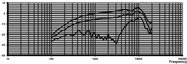
Şek. 1: Frekans yanıtı (Yayıma açısı: 0, 90 ve 180 derece)
