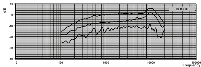
频率响应 (开放角度: 0 度、90 度和 180 度)
