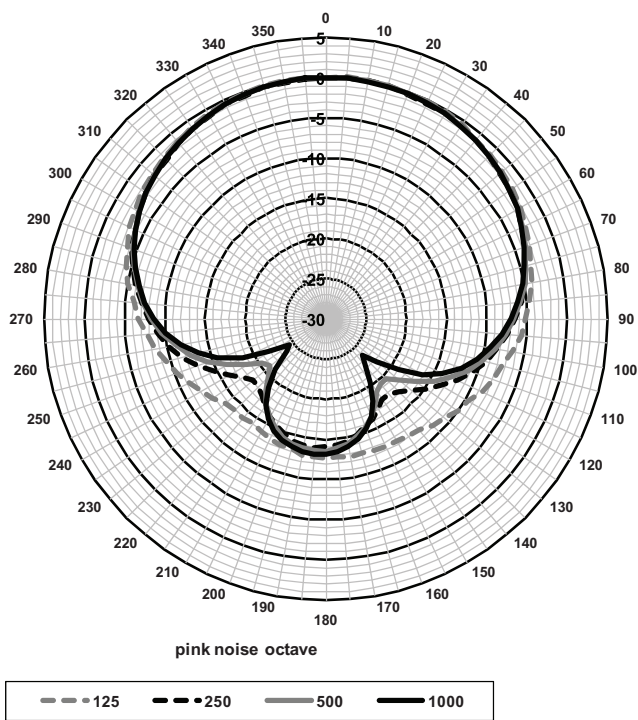
指向性图 (使用粉红噪声测量)
