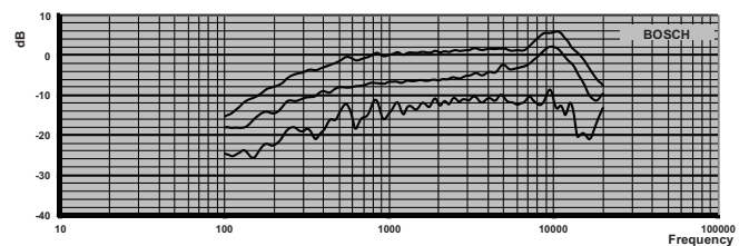
Fig. 1: Risposta in frequenza (angolo di apertura: 0,90 e 180 gradi)
