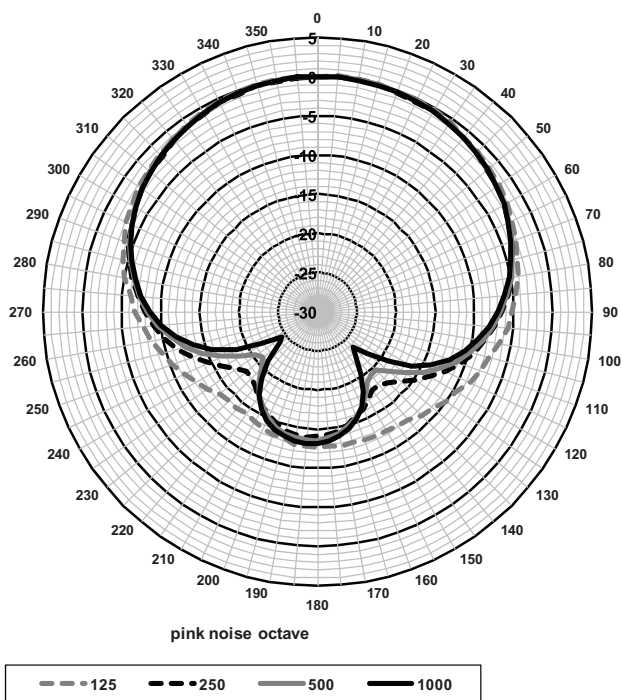
Fig. 2: Schema polare (misurato con il rumore rosa)
