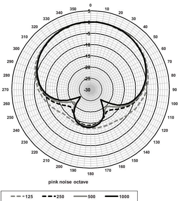
Gbr. 2: Polar diagram (diukur dengan pink noise)
