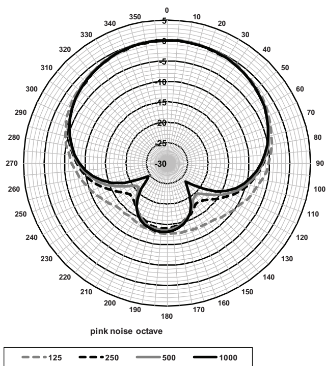
Polárgörbe (rózsaszín zajjal mérve)
