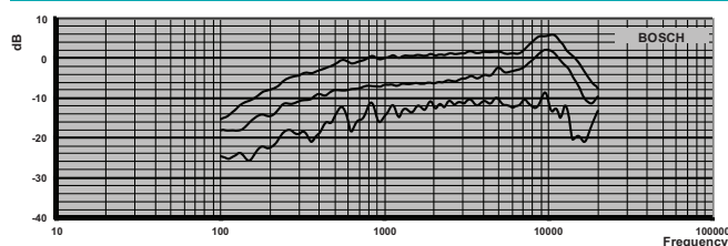
Fig. 1: Réponse en fréquence (angle d'ouverture : 0, 90 et 180 degrés)
