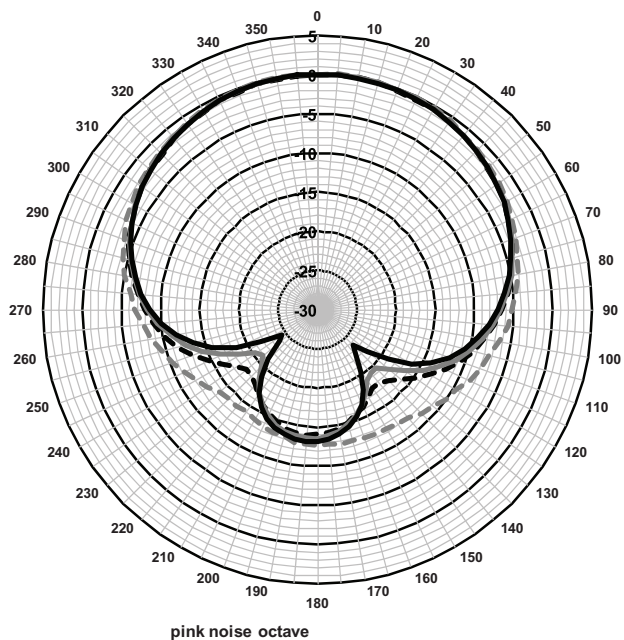
Kuva 2: Suuntakuvio (mitattu vaaleanpunaisella kohinalla)
