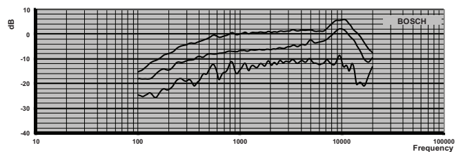
Kuva 1: Taajuusvaste (avauskulma: 0, 90 ja 180 astetta)
