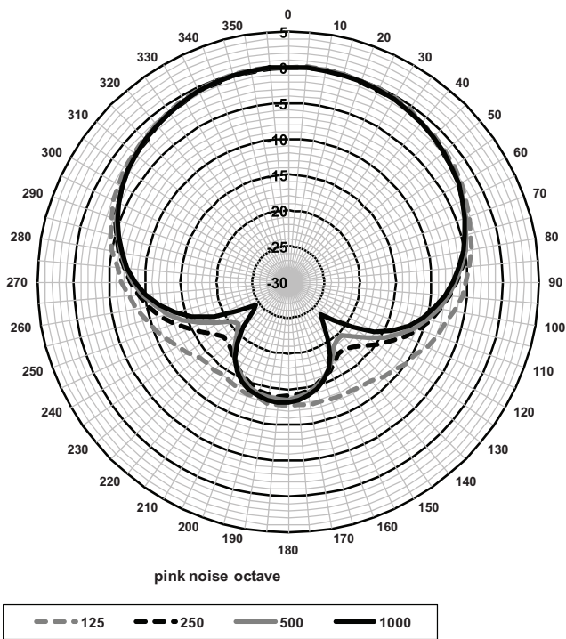
Πολικό διάγραμμα (μέτρηση με ροζ θόρυβο)
