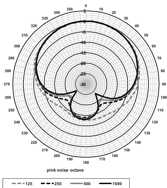
Polární diagram (měřeno s růžovým šumem)
