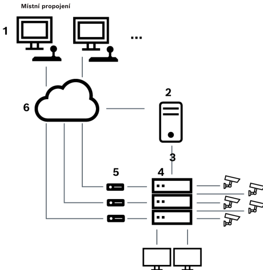
Vyobrazení 6.3: Místní propojení systému Bosch Video Management System s maticovým přepínačem Bosch Allegiant
