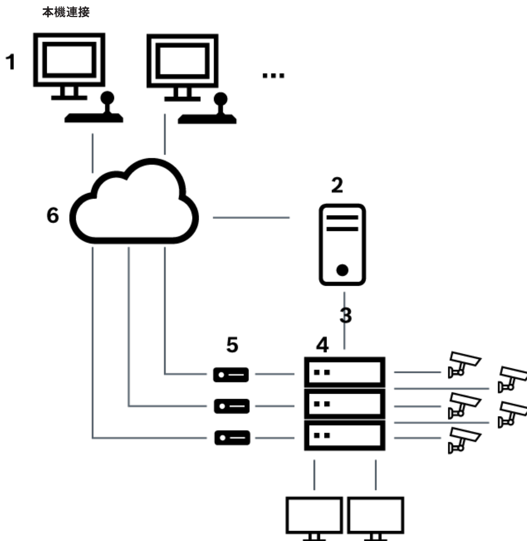
圖片 6.3: Bosch Video Management System 本機連接至 Bosch Allegiant 矩陣切換器
