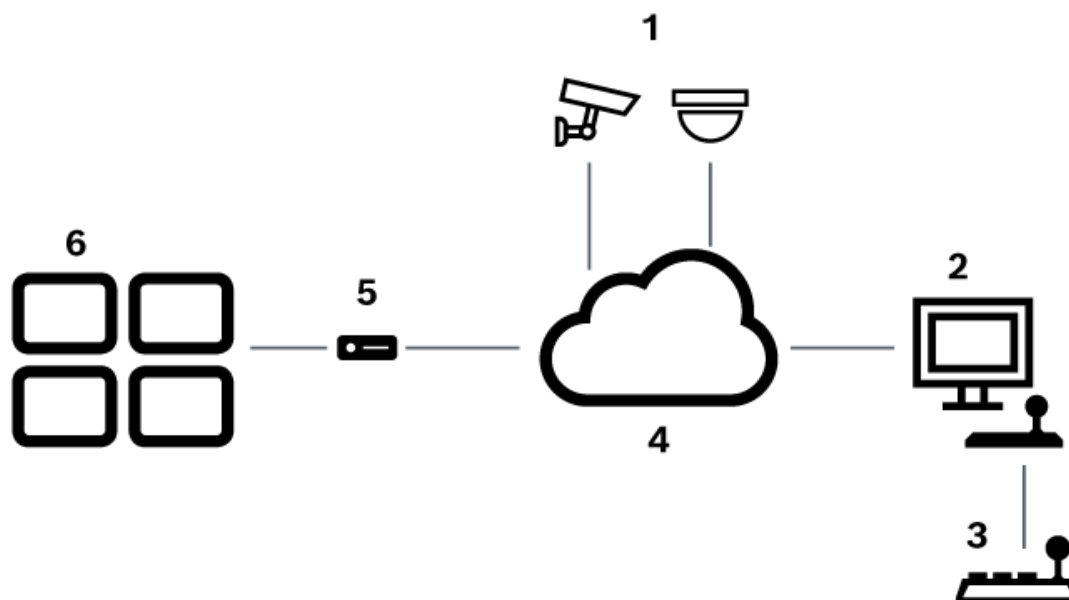
圖片 6.1: 案例 1: Bosch IntuiKey 鍵盤已連接至 Bosch Video Management System 工作站
