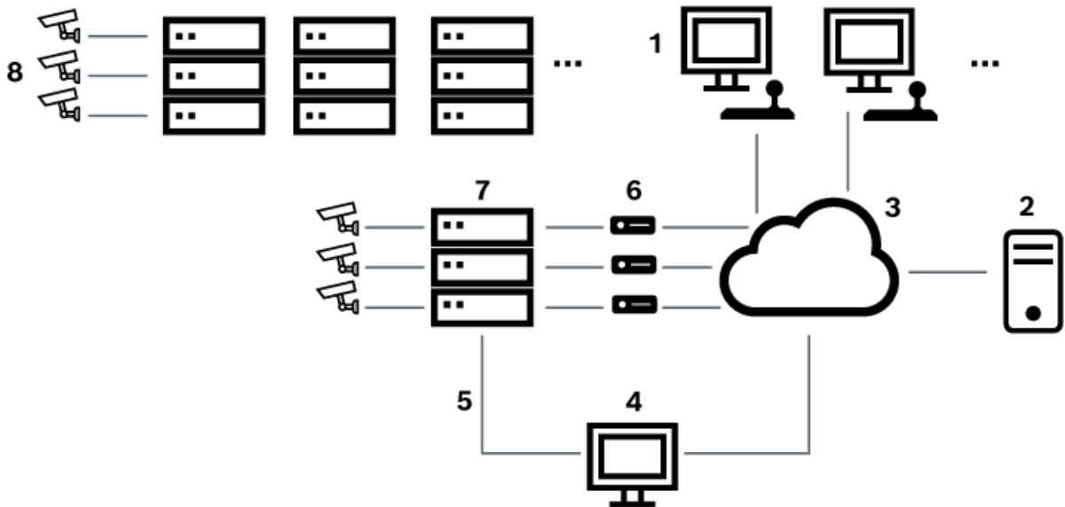
Abbildung 5.5: Mit Satellitenkreuzschienen erweitertes Bosch Allegiant System
