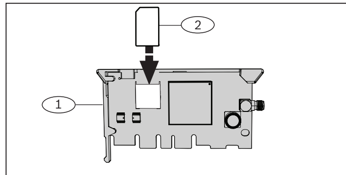
Afbeelding 2.1: De SIM-kaart plaatsen
