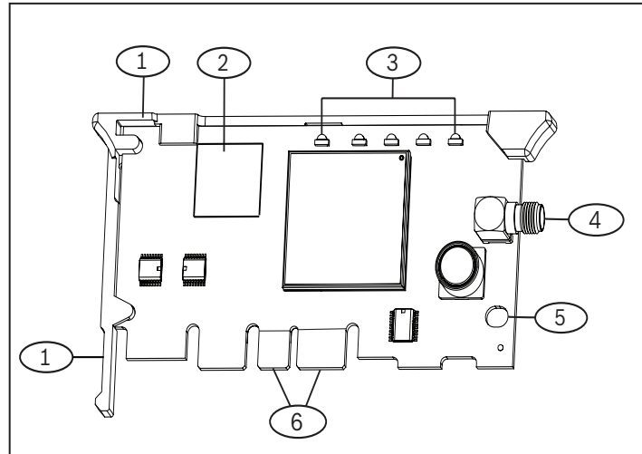
Afbeelding 1.1: Overzicht moederbord
