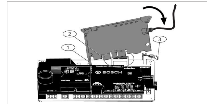
Afbeelding 2.3: De module installeren
