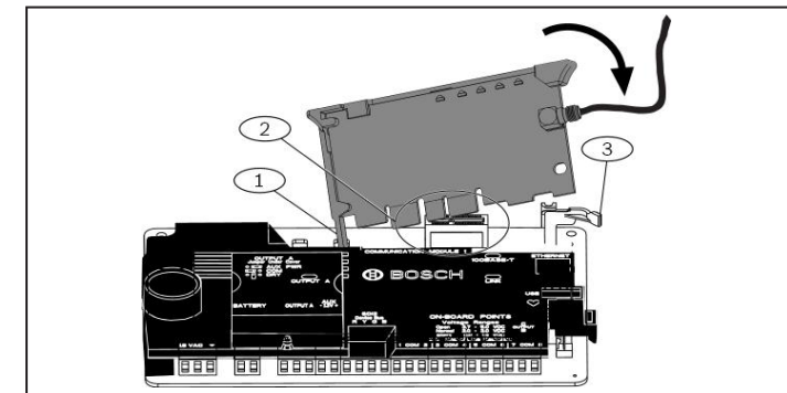
Figure 2.3 : Installation du module
