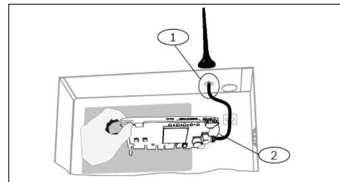
Figure 2.2 : Installation de l'antenne
