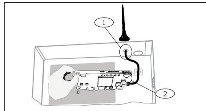
Figura 2.2: Instalación de la antena
