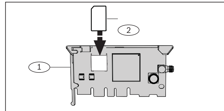
图 2.1: 插入 SIM 卡
