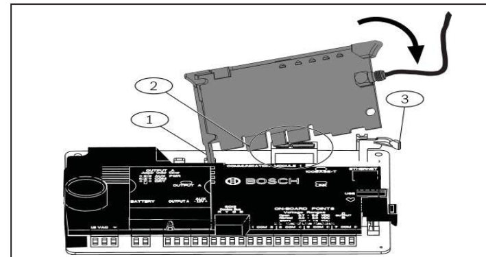
图 2.3: 安装模块
