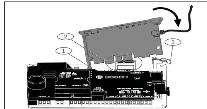
Bild 2.3: Installera modulen
