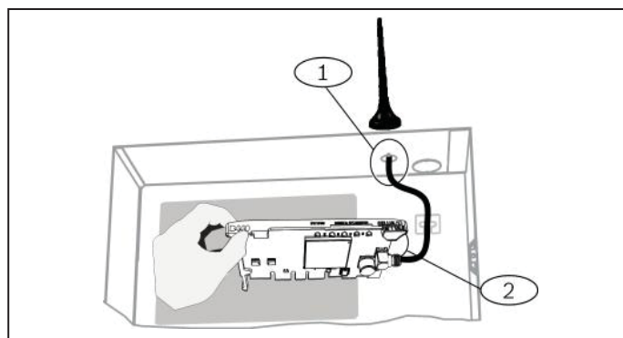
Bild 2.2: Installera antennen
