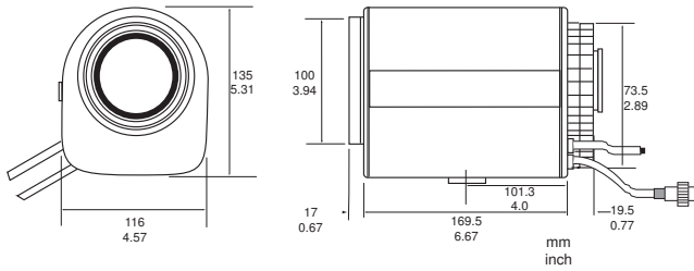
Mått LTC 3293/40 och LTC 3293/50
