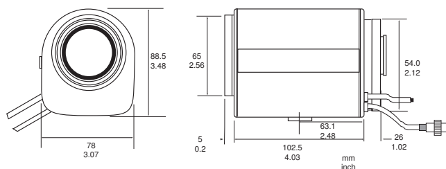
Rozměry objektivů LTC 3293/20 a LTC 3293/30
