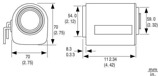
Rozměry objektivu LTC 3384/21
