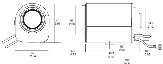
Rozměry objektivu LTC 3283/40
