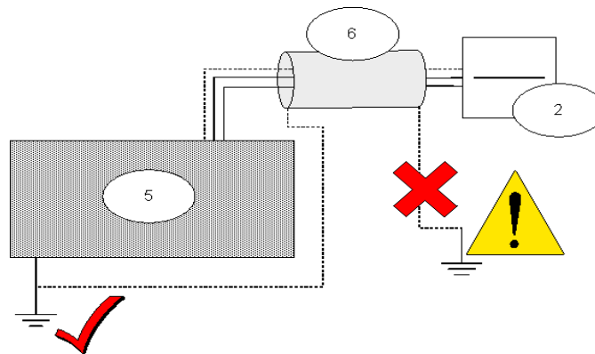
Bild 4.3 Vermeidung von Erdschleifen
