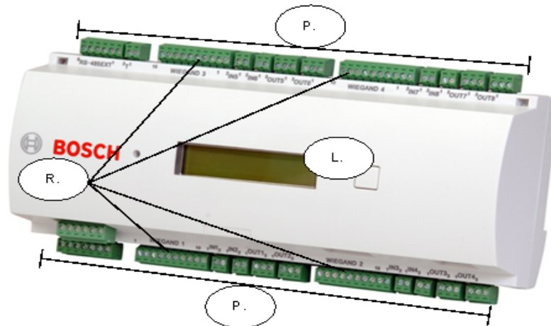
Bild 3.4 AMC2-Zutrittskontrollzentrale
