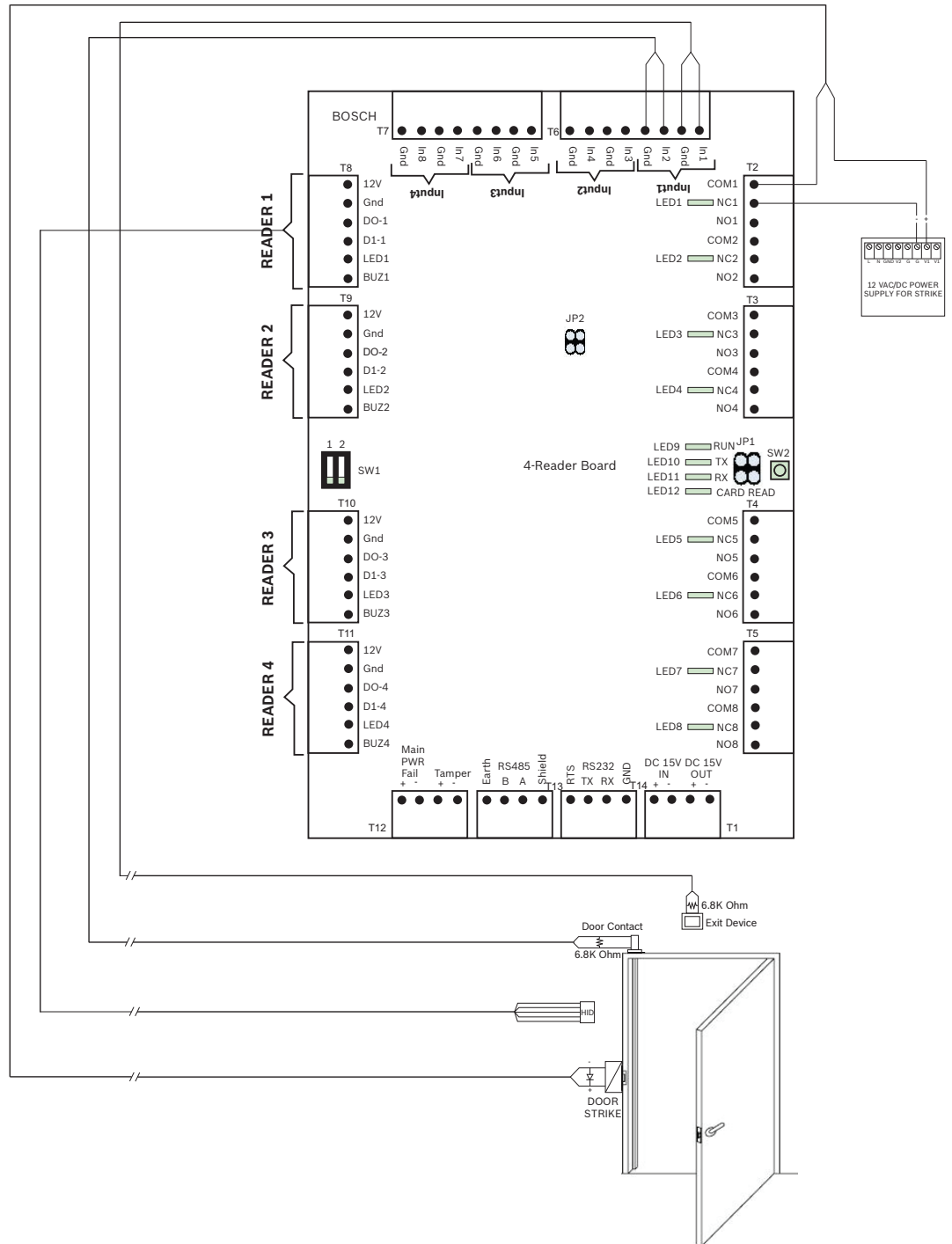
Bild 4.5 AEC2.1-Anschlüsse für eine Tür
