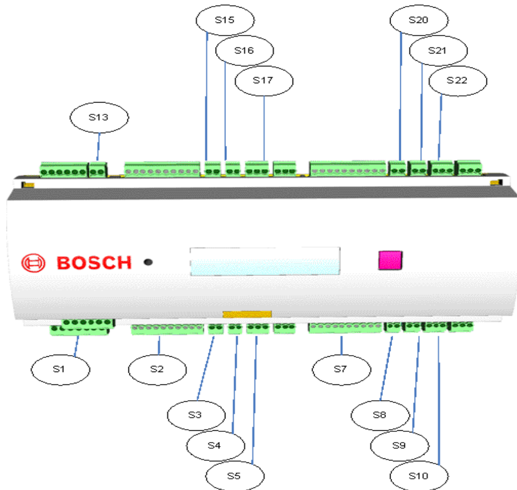
Bild 3.5 Die im Beispiel der 4-Raum-Arztpraxis verwendeten AMC2-Anschlüsse
