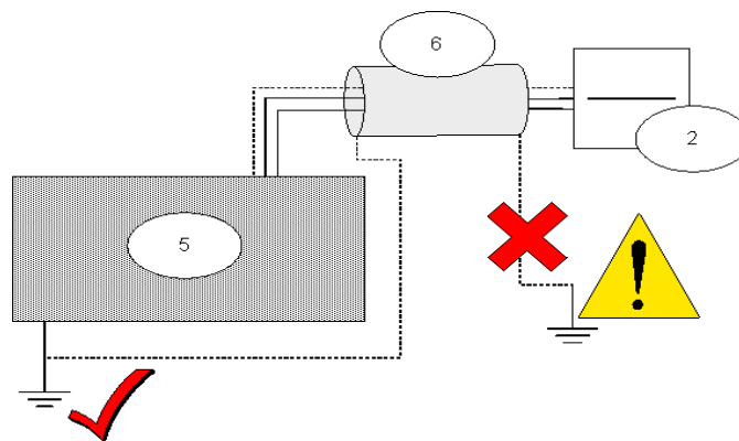
Bild 3.3 Vermeidung von Erdschleifen
