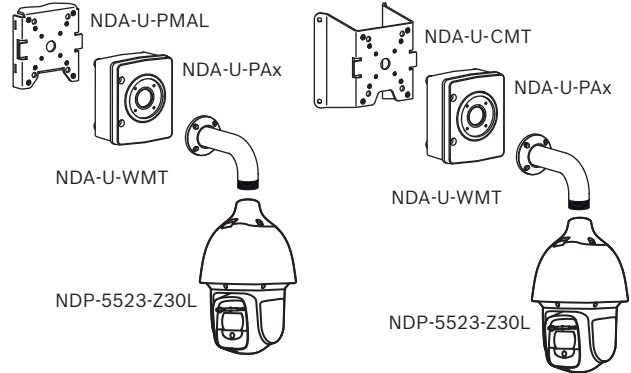
Şek. 2: Direğe montaj düzeneği (IP66); köşeye montaj düzeneği (IP66)
