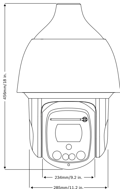
寸法図
