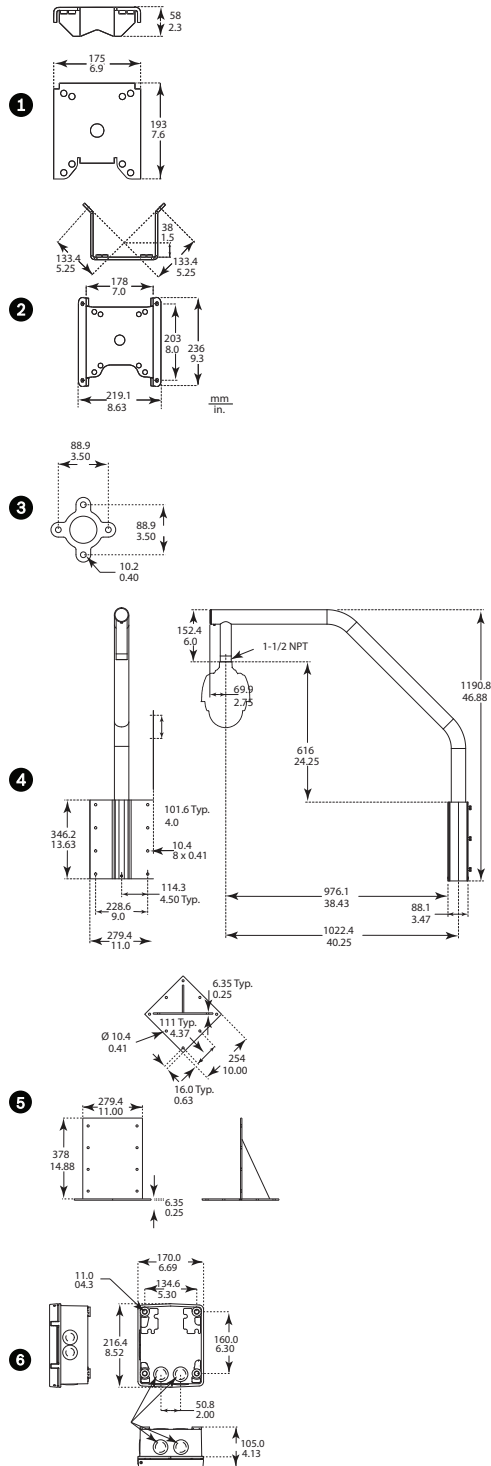
Fig. 2: AutoDome Série 7000 Suportes opcionais
