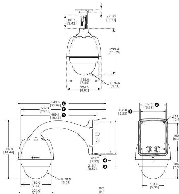
Fig. 1: Dimensões, suporte para tubulação AUTODOME7000, suporte suspenso
