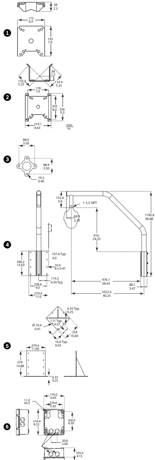
Rys. 2: Mocowania opcjonalne z serii AUTODOME 7000
