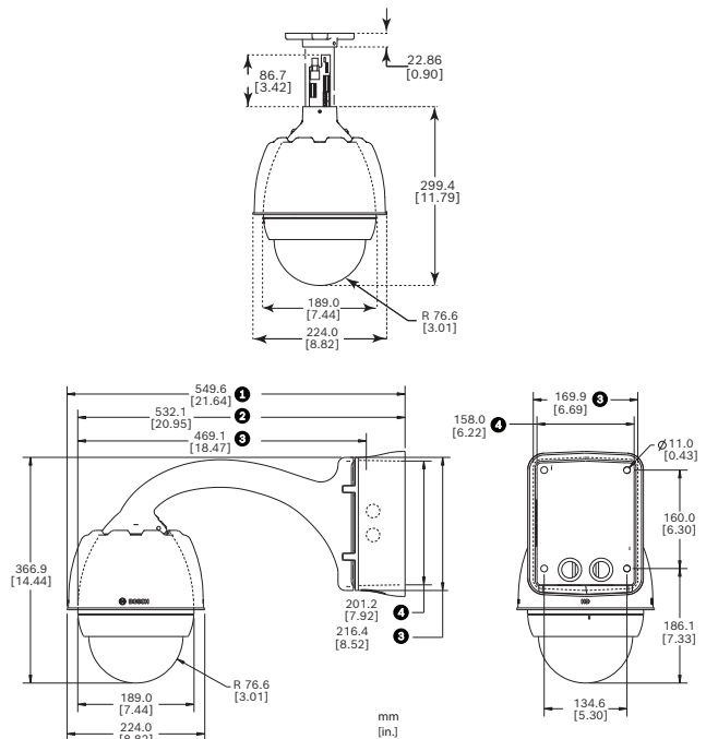
Fig. 1: Dimensions, montage suspendu plafond AUTODOME7000
