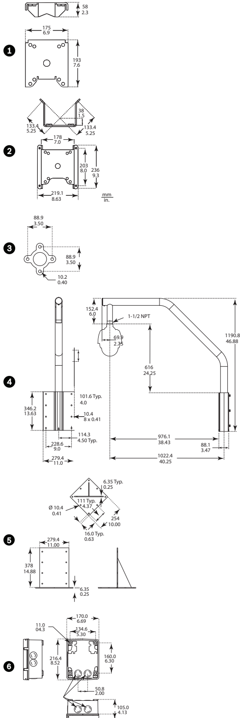
Fig. 2: Montages en option pour AUTODOME 7000 series
