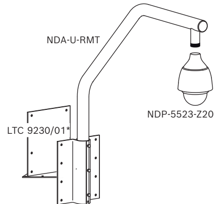
圖 4: 屋頂基座安裝 (IP66)
