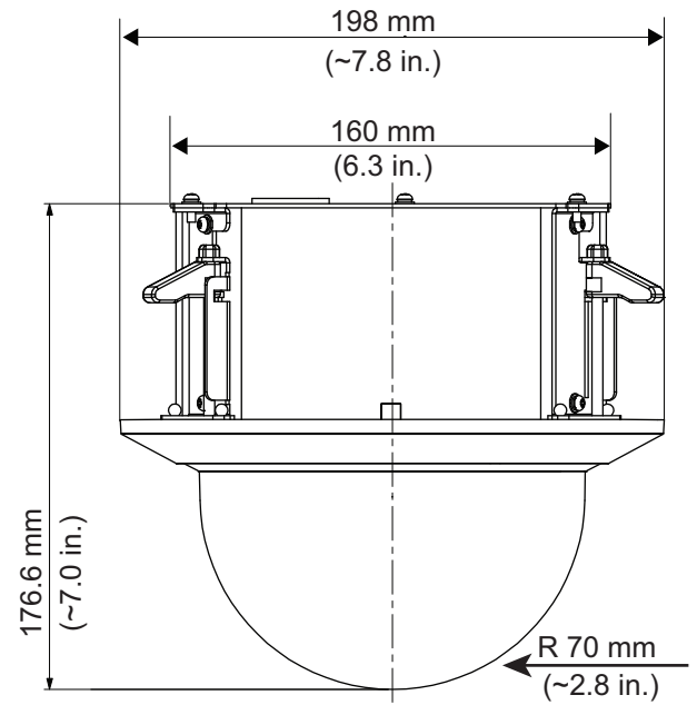
圖 6: 天花板掛架機型
