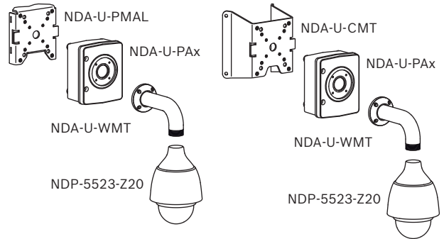
圖 3: 孔洞基座安裝；轉角掛架 (IP66)
