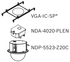
图片 5: 天花板安装
