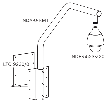
图片 4: 屋顶安装(IP66)
