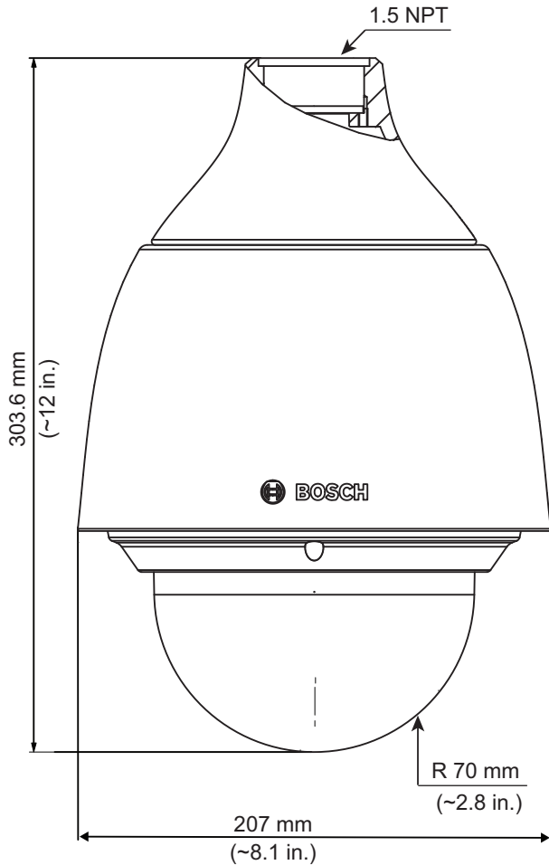
图片 7: 悬吊式型号
