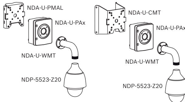
图片 3: 立杆安装(IP66); 墙角安装(IP66)
