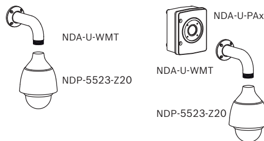
图片 1: 墙壁安装; 配备监控电源盒(IP66)的墙壁安装
