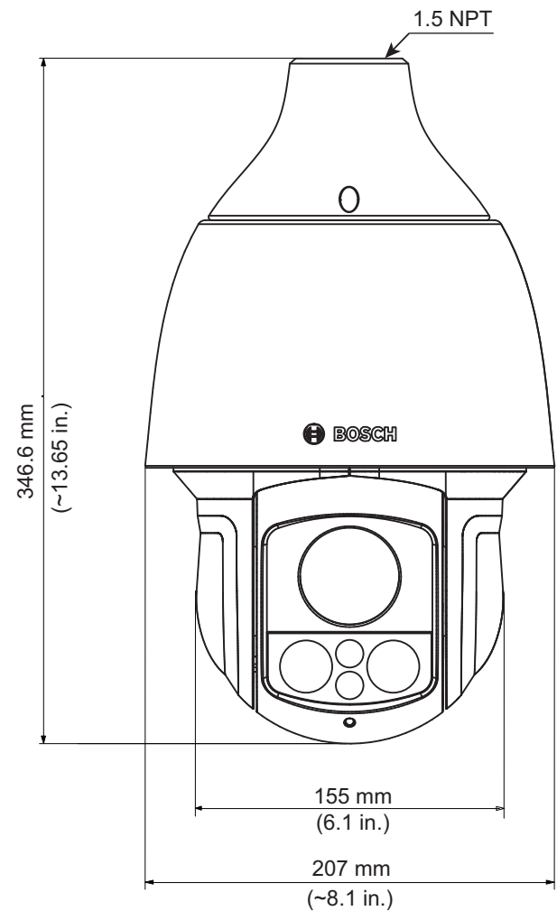
尺寸图
