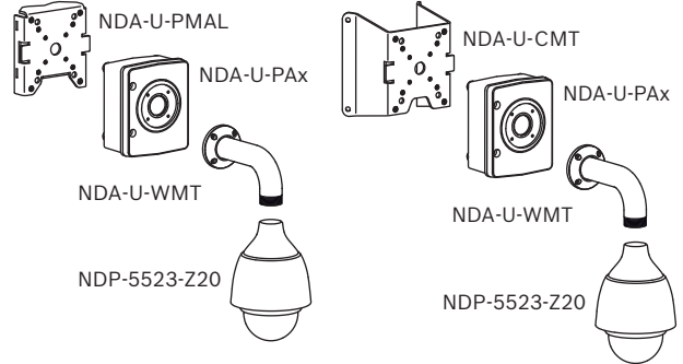
Şek. 3: Direğe montaj düzeneği (IP66); Köşeye montaj düzeneği (IP66)
