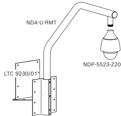
Şek. 3: Direğe montaj düzeneği (IP66); Köşeye montaj düzeneği (IP66)
