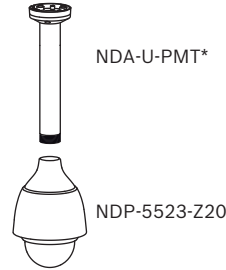
Şek. 2: Askılı boruya montaj düzeneği *NDA-U-PMTE: İsteğe bağlı 50 cm/20 inç uzatma borusu
