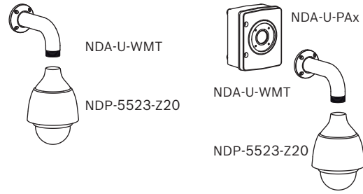
Şek. 1: Duvara montaj düzeneği; Gözetim kabinine sahip duvara montaj düzeneği (IP66)
