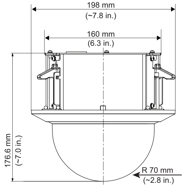
Şek. 6: Asma tavan modeli
