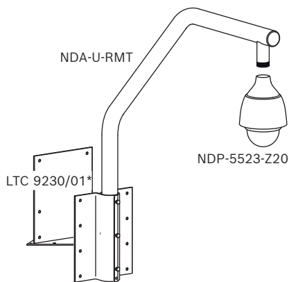
Рис. 3: Монтаж на столб (IP66); кронштейн для установки в угол (IP66)
