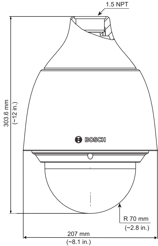
Рис. 7: Подвесная модель
