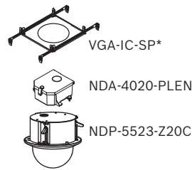
Рис. 5: Монтаж в потолок *Дополнительно Дополнительные варианты монтажа см. в документе Краткое руководство по выбору изделий: виды монтажа модульных камер и дополнительные принадлежности.
