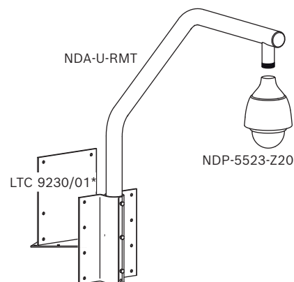
Afb. 4: Dakmontage (IP66)
