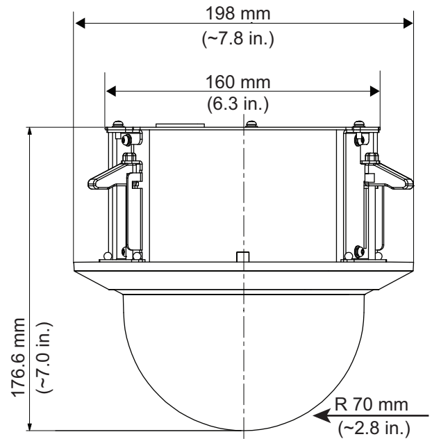
Afb. 6: Plafondinbouw
