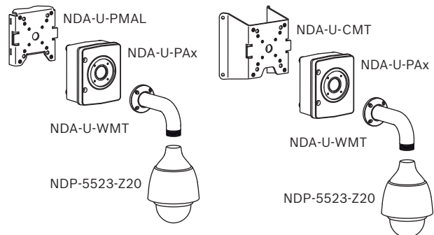
Afb. 3: Mastmontage (IP66); hoekmontage (IP66)
