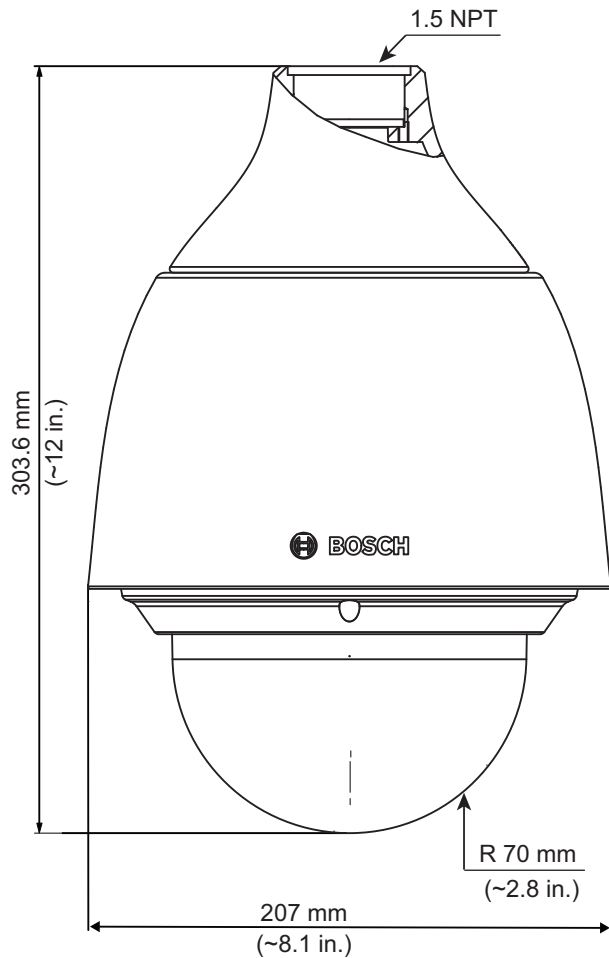
Afb. 7: Boogmodel
