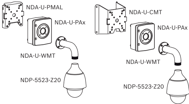
図. 3: ポール マウント (IP66)、コーナー マウント (IP66)
