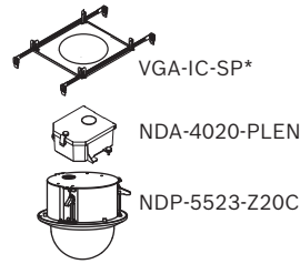
図. 5: 天井埋め込み型マウント
