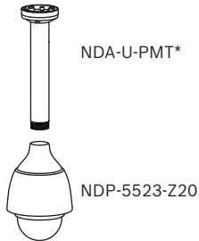
図. 2: 吊り下げ型パイプマウント NDA-U-PMTE: オプションの 50 cm / 20 in 延長パイプ
