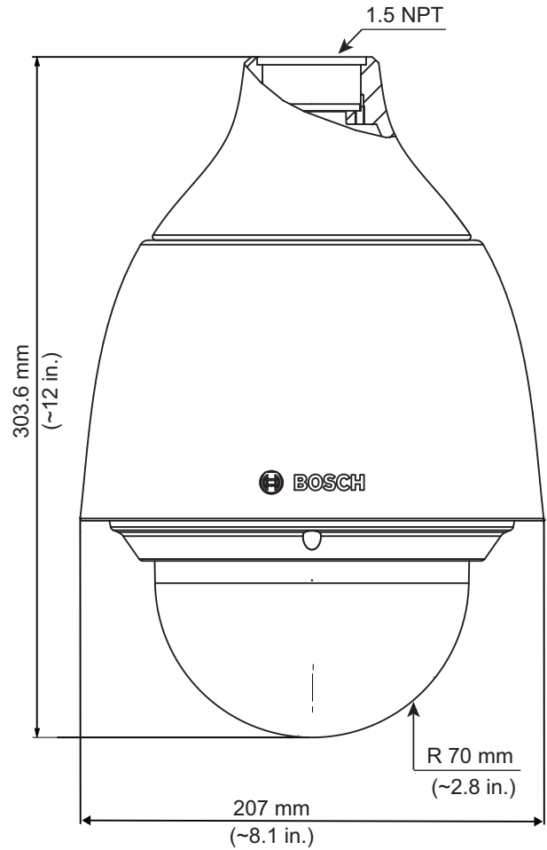
図. 7: 吊り下げ型モデル
