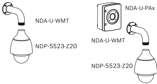
図. 1: ウォール マウント: 監視キャビネット付きウォールマウント (IP66)
