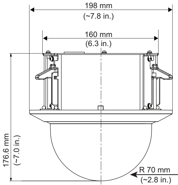
図. 6: 天井埋め込み型モデル
