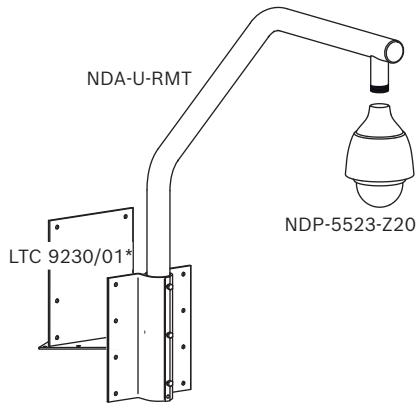
図. 4: ルーフ マウント (IP66) *フラット ルーフ取付け用オプション
