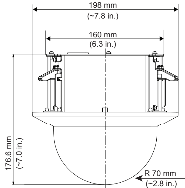
Рис. 2: Потолочная модель
