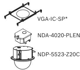
Рис. 1: Монтаж в потолок *Дополнительно
