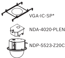
Afb. 1: Plafondbouw *Optioneel
