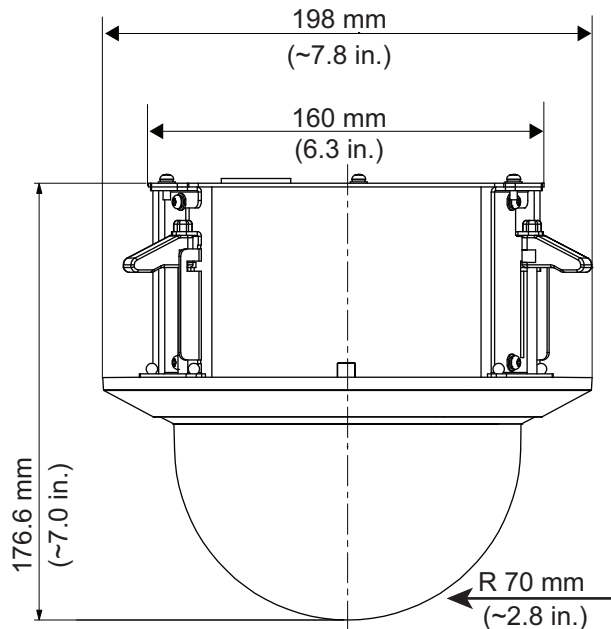
Afb. 2: Plafondbouw
