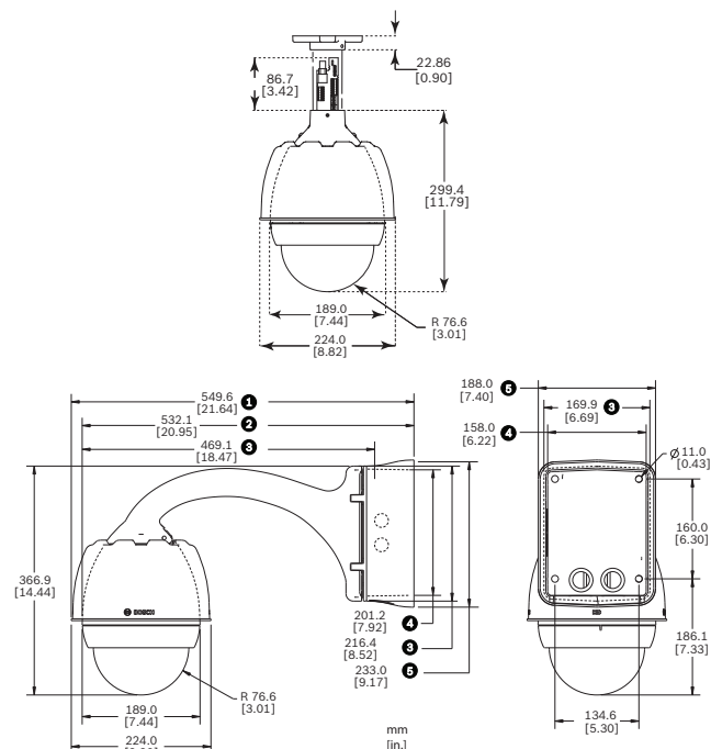
AutoDome Série 7000 Tubo, suportes pendentes
