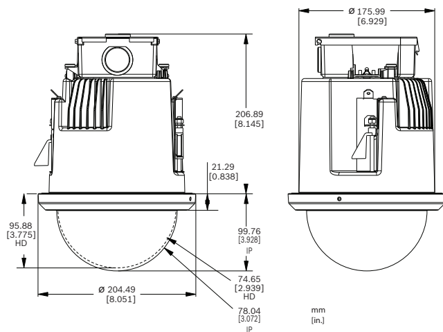
AutoDome Série 7000 encastrada no teto
