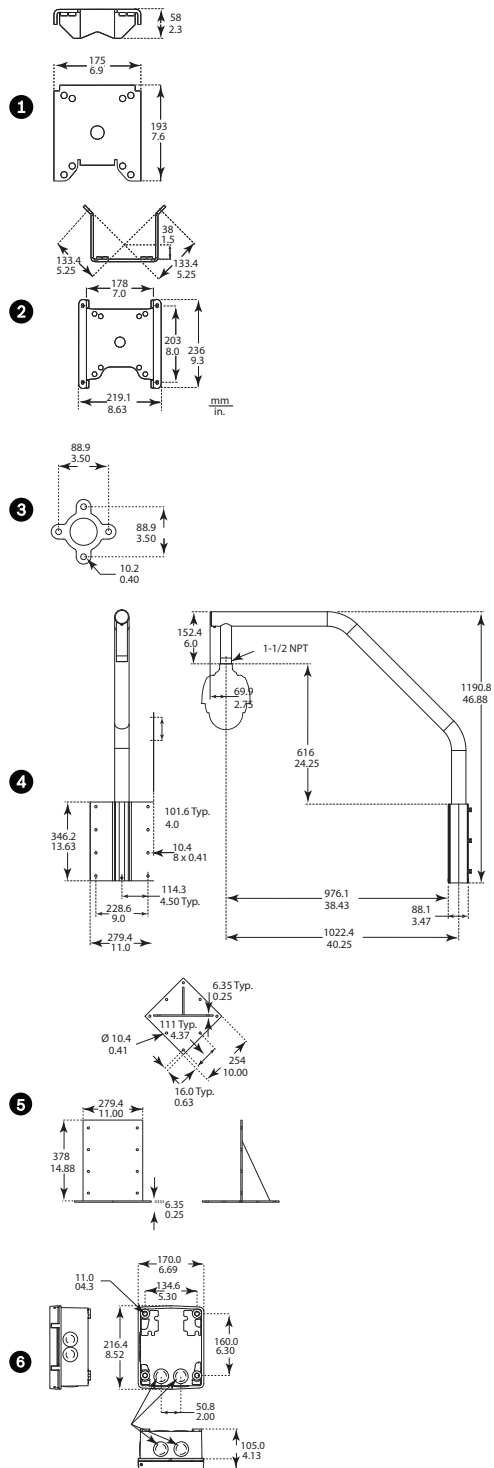
Rys. 3: Mocowania opcjonalne z serii AUTODOME 7000
