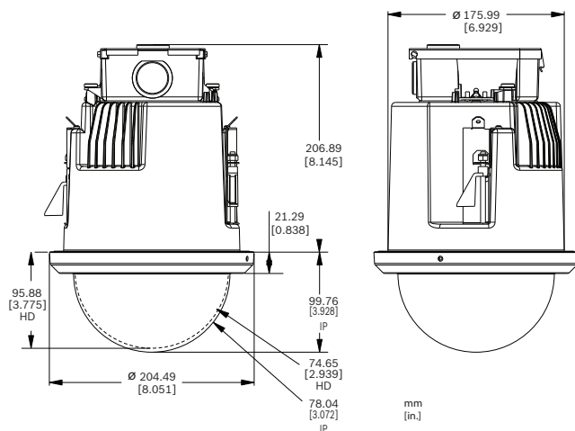
Serie AUTODOME 7000 a incasso
