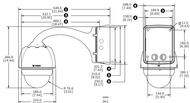
Staffe pendente e per tubo serie AUTODOME 7000
