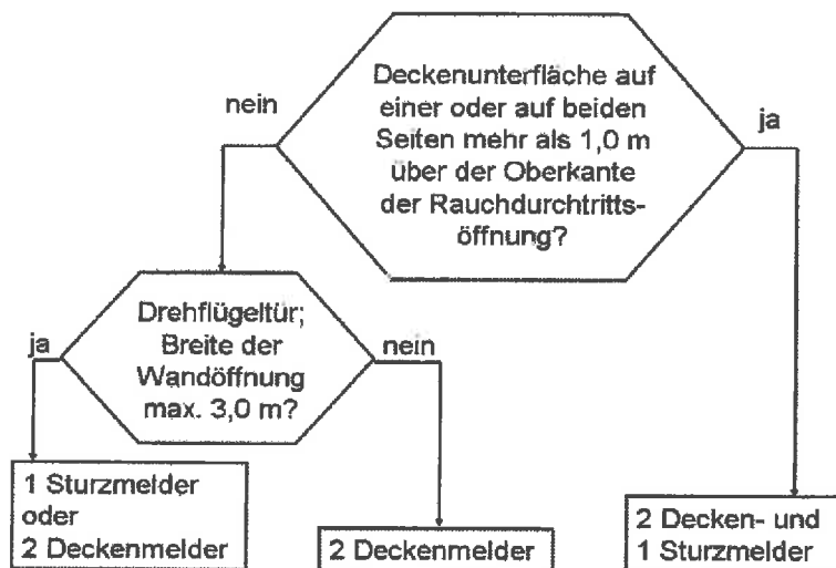
Bild 3: Entscheidungsdiagramm
